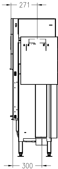
Horizontalschnitt M~1:10
