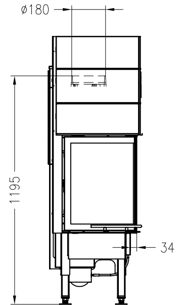
Seitenansicht M~1:20
